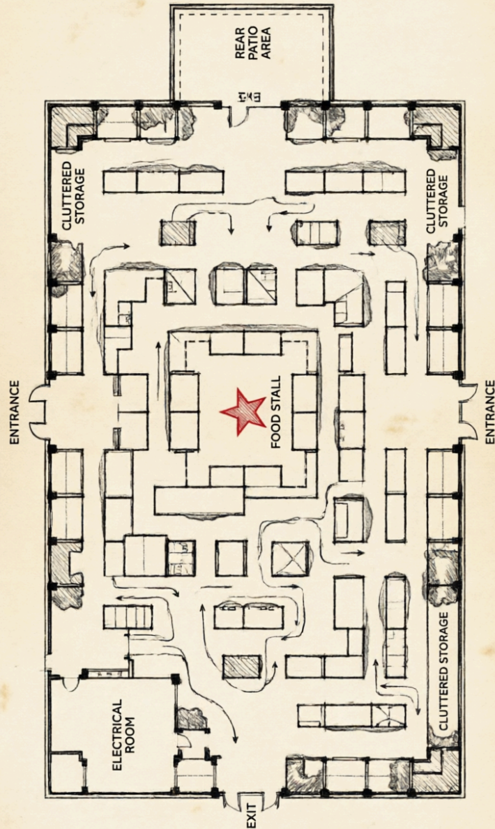
Architectural floor plan map of Galpón 1 (Sopaipillas El Edén)
